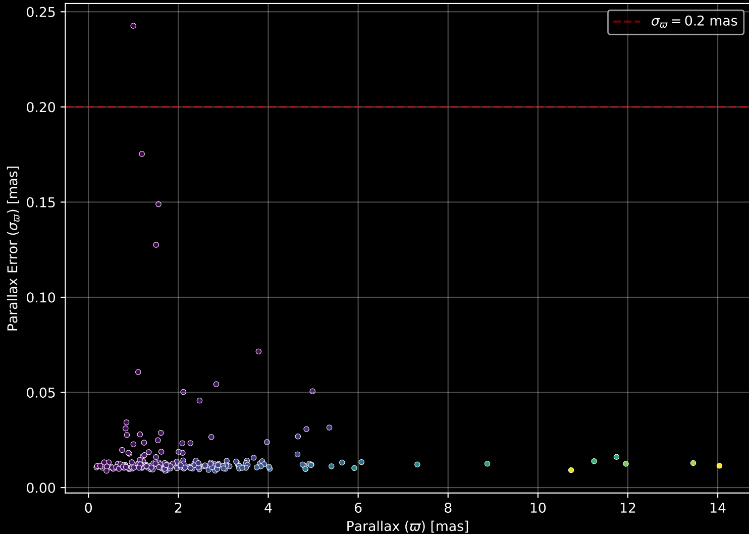
GALAH DR4 Field: [7172] Parallax Quality (n= 200)
