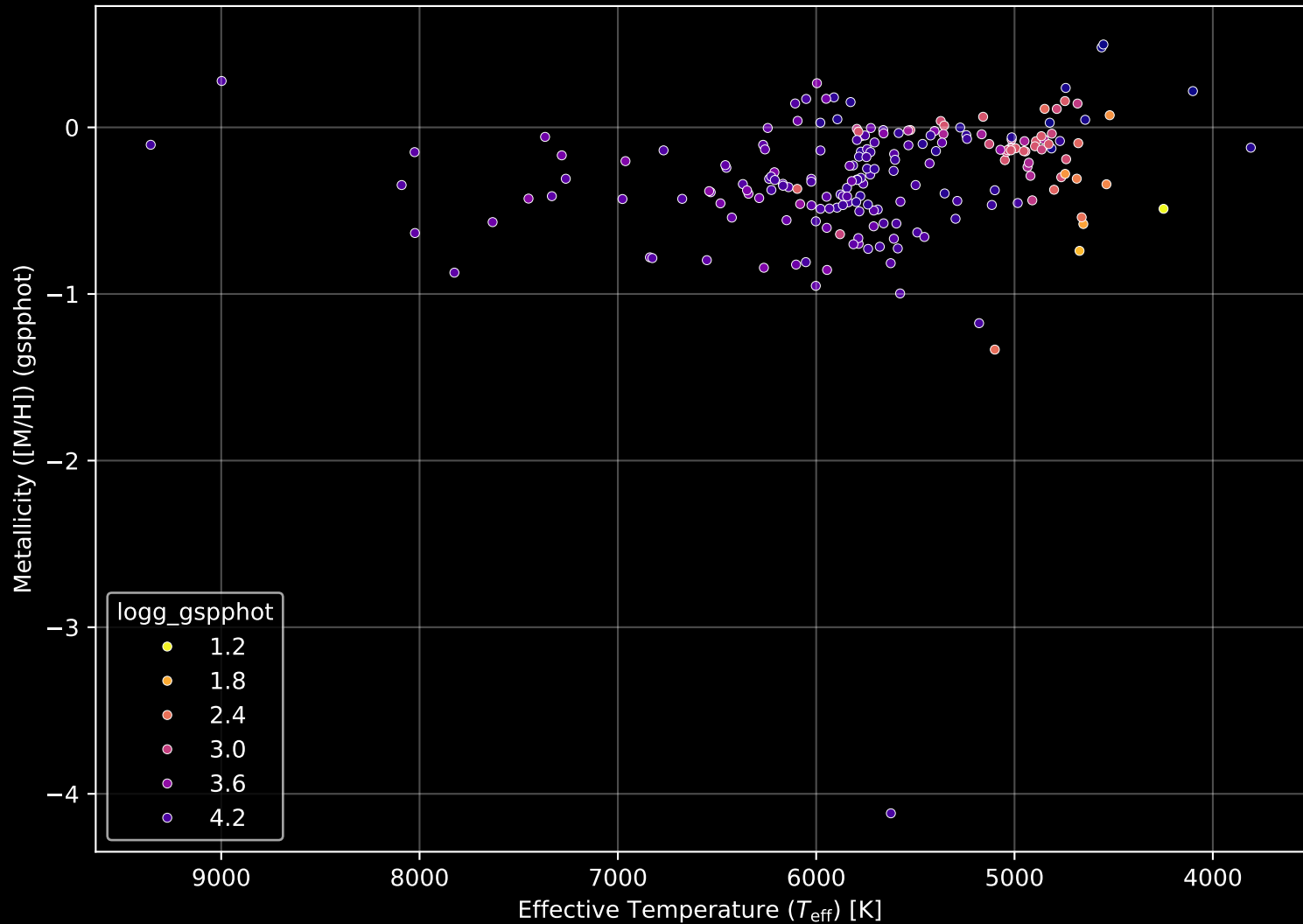
GALAH DR4 Field: [7172] Stellar Population Parameters (n= 200)
