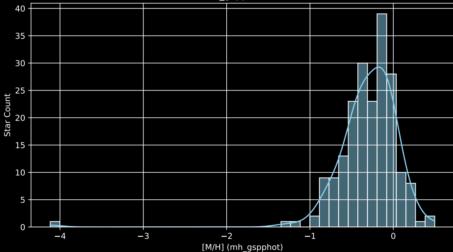
GALAH DR4 Field: [7172] [M/H] (mh_gspphot) (n= 200)
