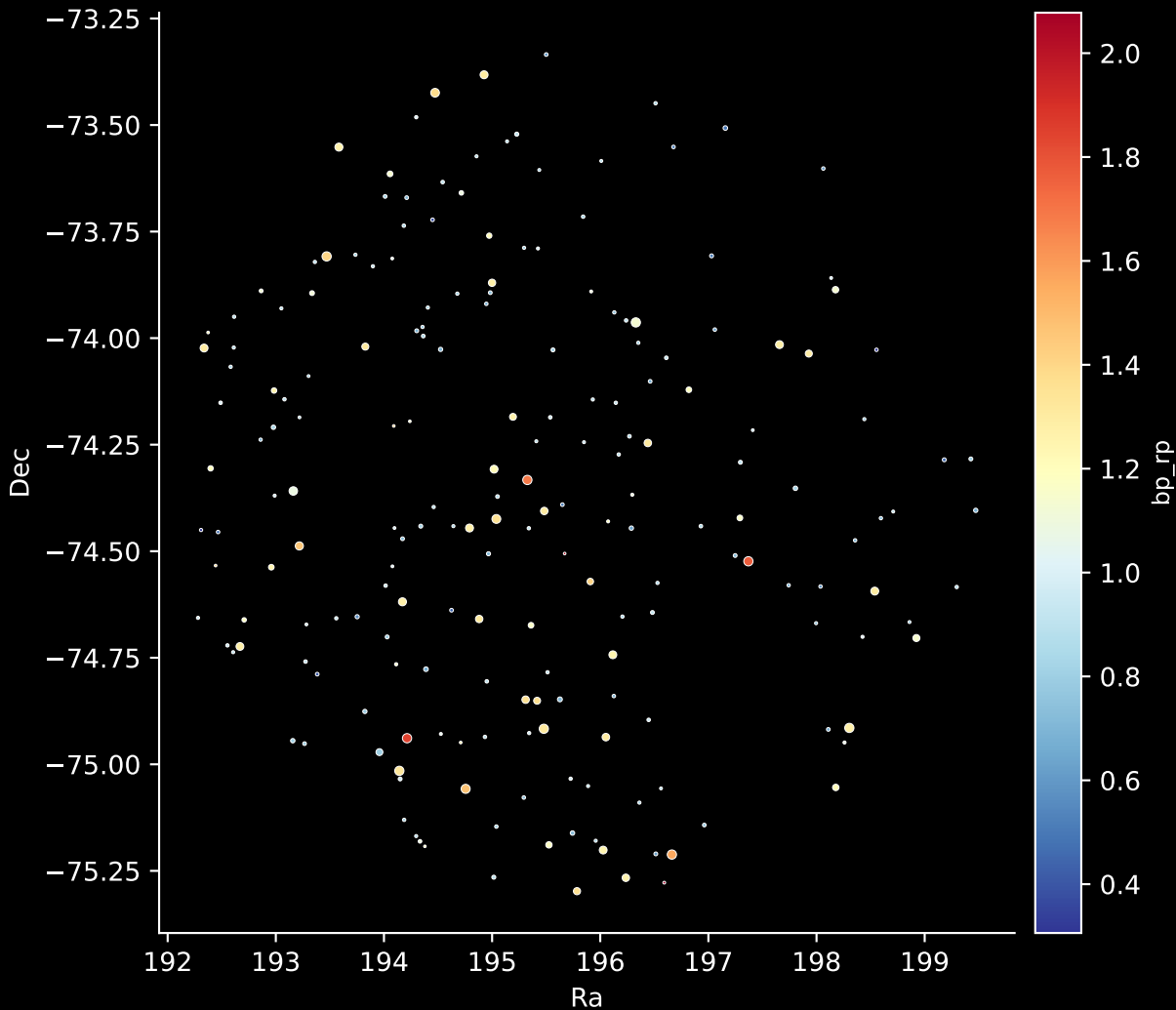
GALAH DR4 Field: [7172] Stars: 200
